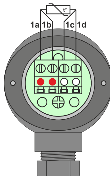
LINIA 4-PRZEWODOWA
