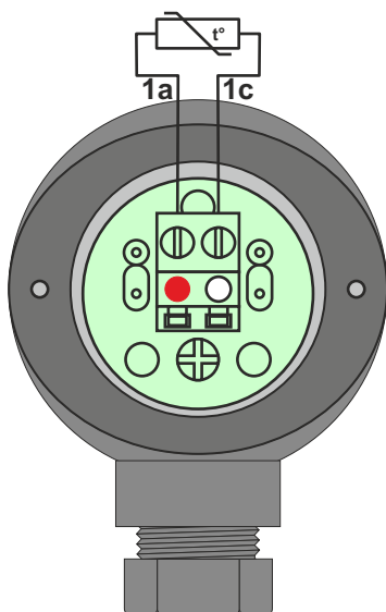
LINIA 2-PRZEWODOWA
