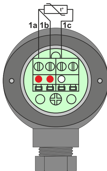
LINIA 3-PRZEWODOWA
