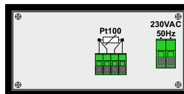
płyta tylnia (połączenia)
